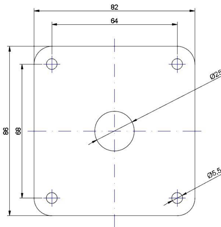
Рисунок 3. Присоединительные размеры ДУТ.
