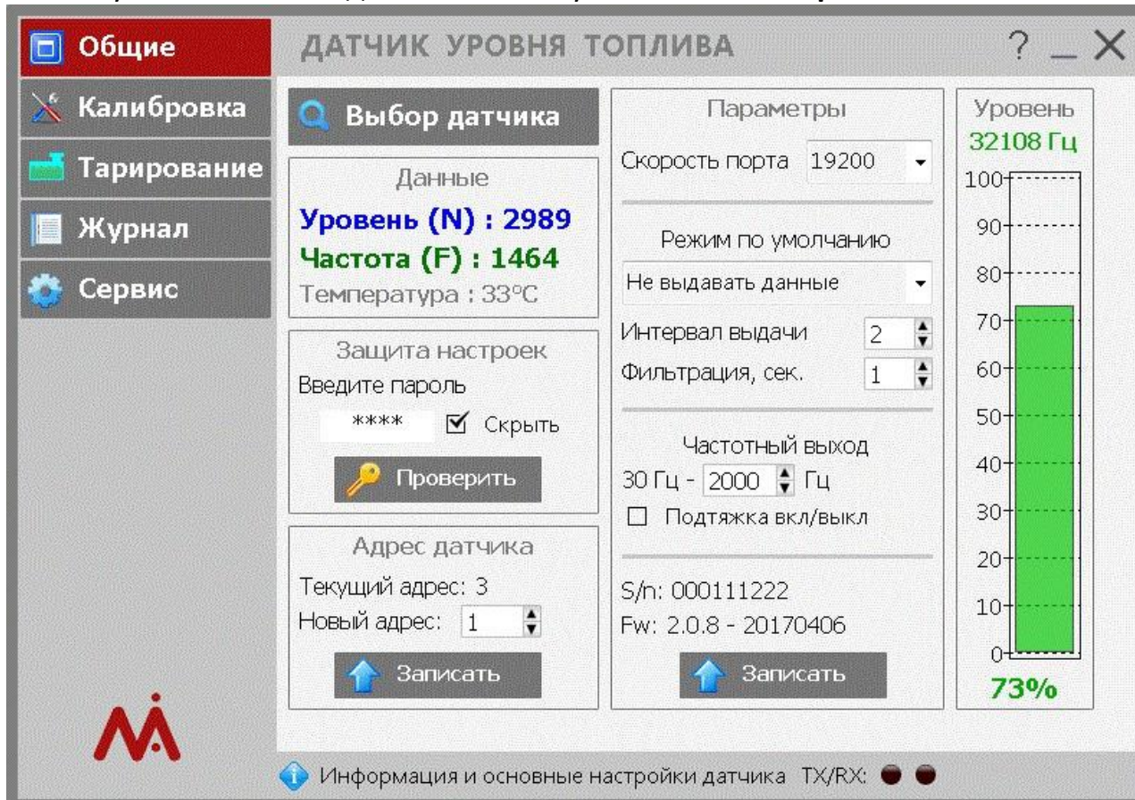
Рисунок 8. Главное окно программы-конфигуратора
