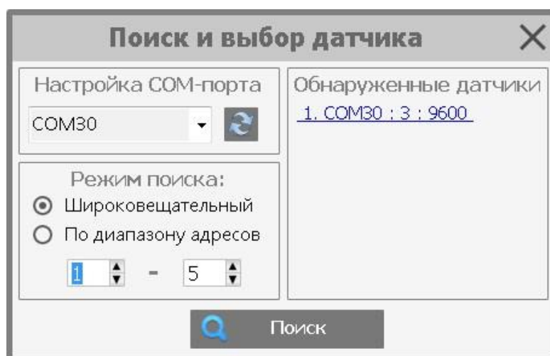
Рисунок 9. Окно «Поиск и выбор датчика»
