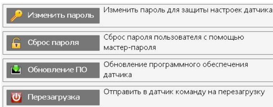
Рисунок 103. Меню «Сервис».
