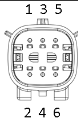
Рисунок 7. Нумерация контактов в разъеме ДУТ.
